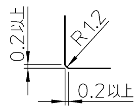
X部詳細
